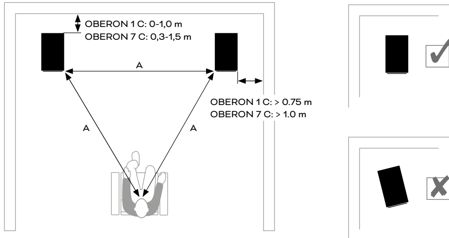
DIAGRAMA 3A - CONFIGURACIÓN STEREO DALI OBERON 1 C & 7 C
