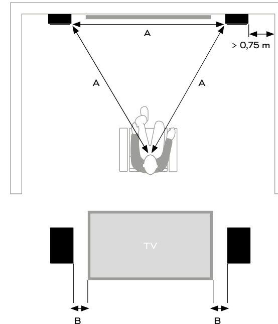
DIAGRAMA 3B - CONFIGURACIÓN STEREO DALI OBERON ON-WALL C
